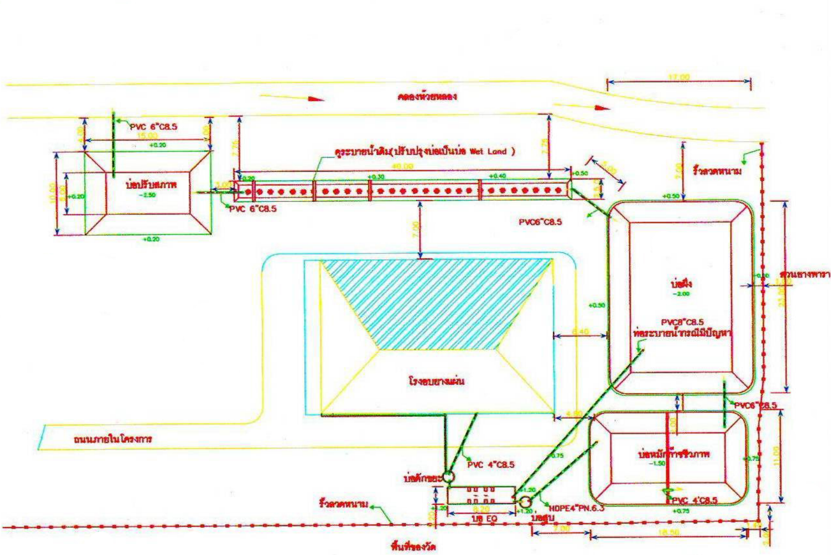
แผนผังพื้นที่สหกรณ์กองทุนสวนยางของหลังทำการปรับปรุง SCALE 1: 300
