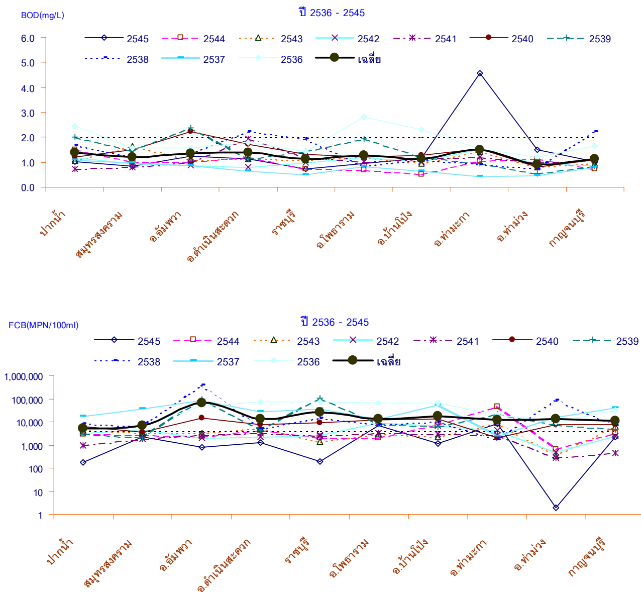
รูปที่ 4 คุณภาพน้ำแม่น้ำแม่กลอง ปี 2536 - 2545
