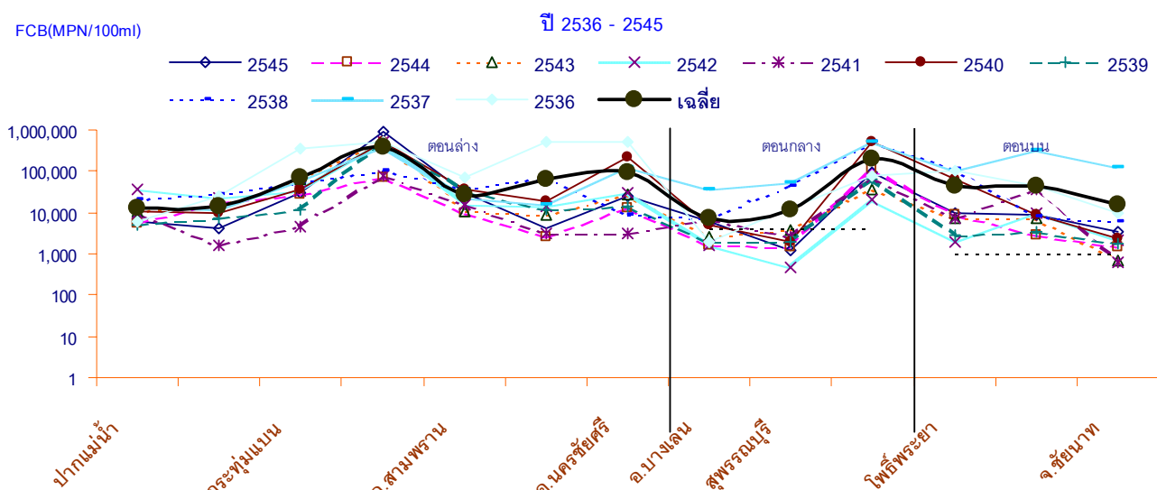
รูปที่ 2 คุณภาพน้ำแม่น้ำท่าจีน ปี 2536 - 2545
